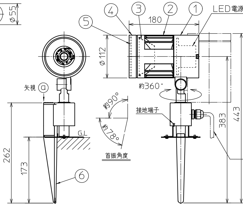
○ 矢視図
