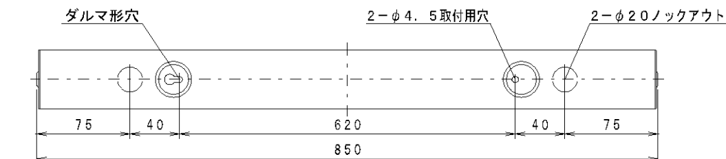
上向き取付の場合
