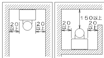
下向き取付の場合
