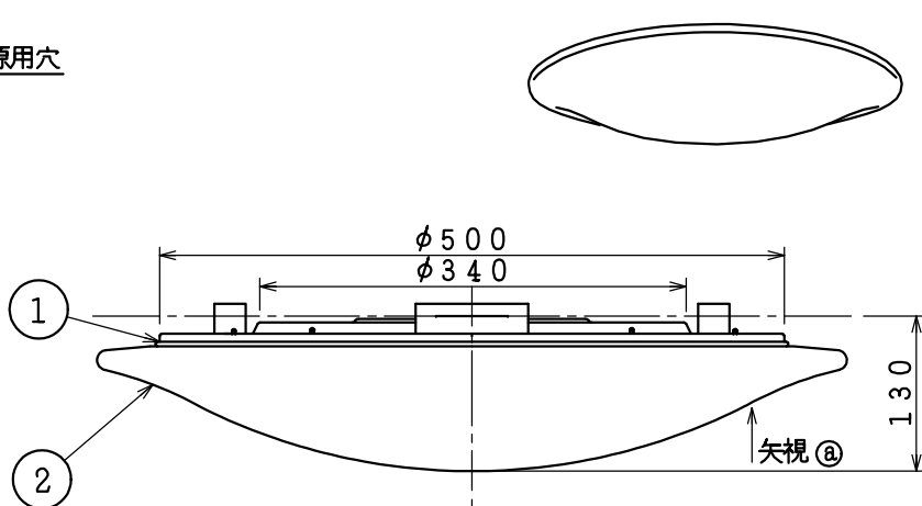
取付寸法 (矢視 a)
