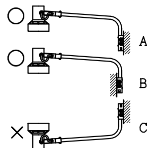
取付方向可否図
