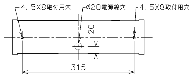
天井取付寸法 (矢視 ㊹)
