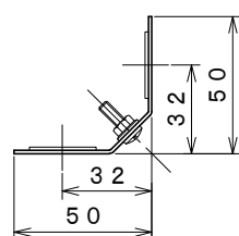
取付寸法 (矢視 a)
