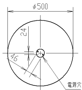
取付寸法（矢視 ①）
