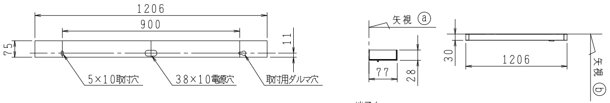
取付寸法 直付の場合(矢視 ㉔)
