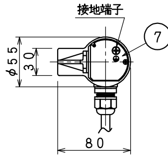
取付寸法（矢视图 ⑧）
