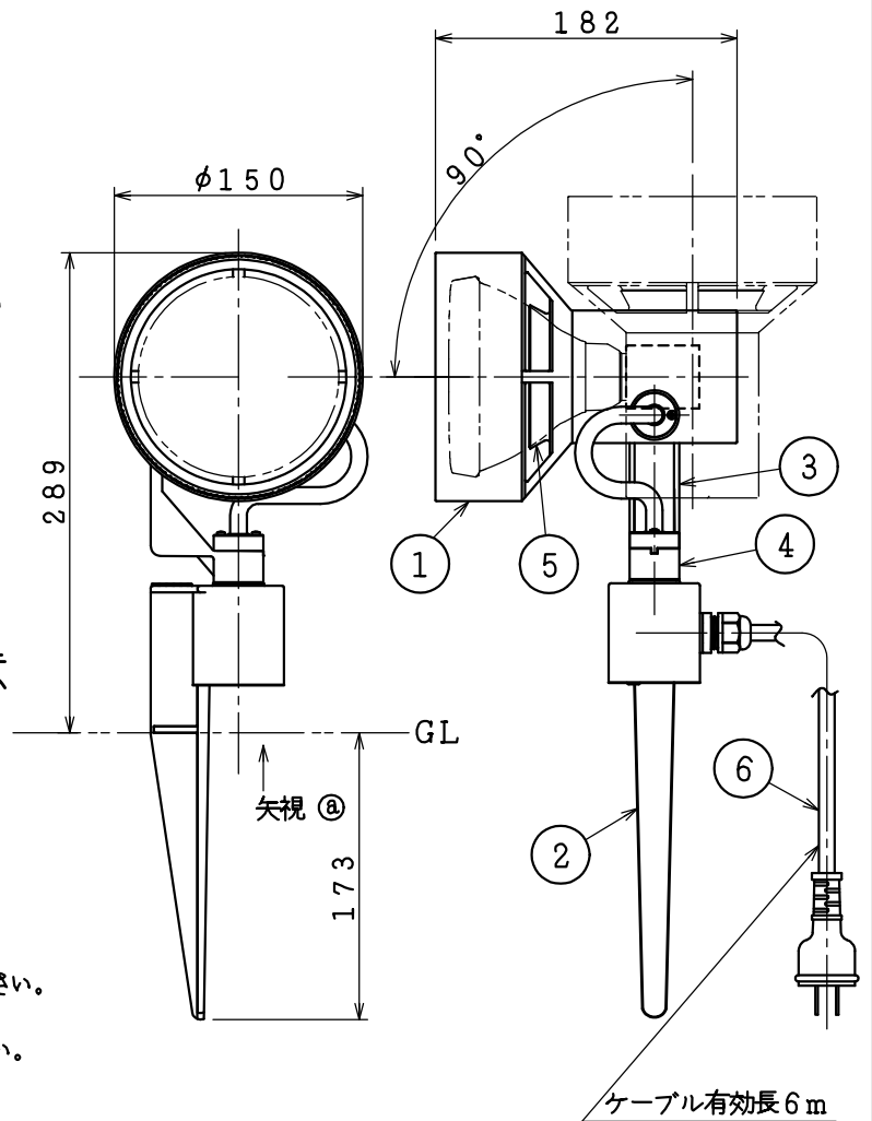
灯具可動範囲
