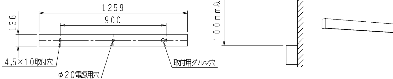
取付寸法（矢視 ②）
