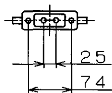
取付寸法（矢視④）
