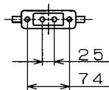
取付寸法（矢視②）
