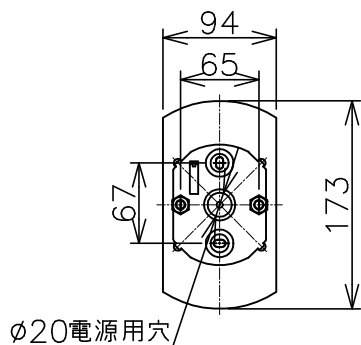
取付寸法 (矢視 ①)
