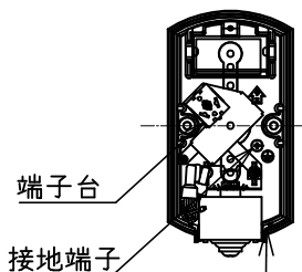
取付寸法 (矢視 ①)
