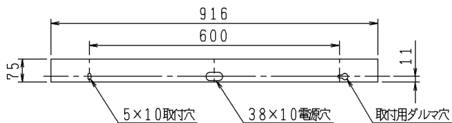
取付寸法 直付の場合（矢視 ㊹）
