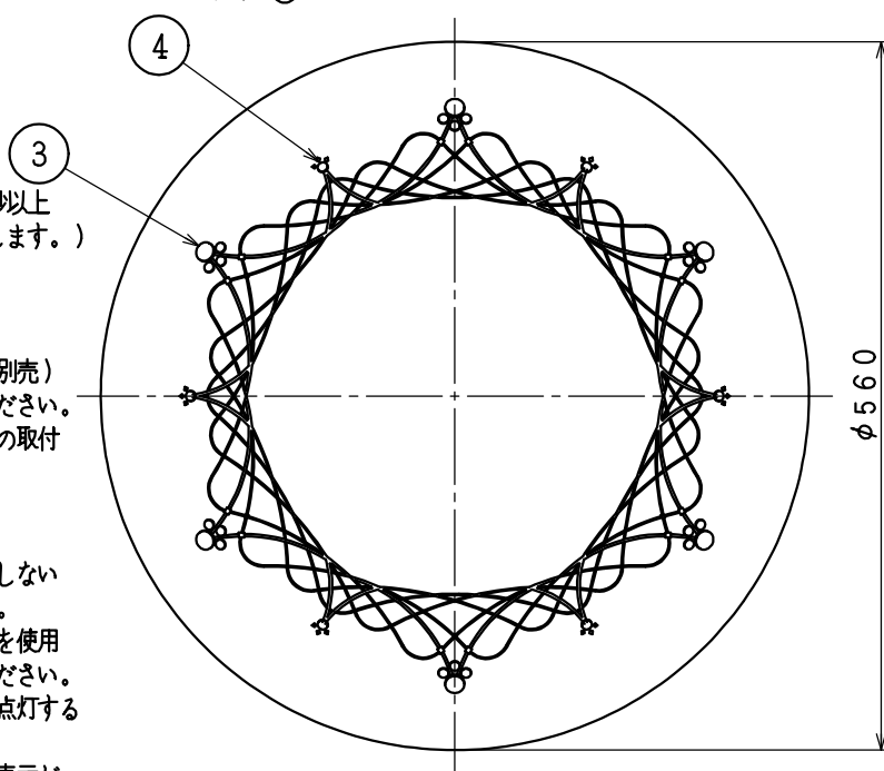
矢視 a
