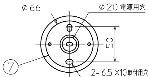
取付寸法(矢視A)
