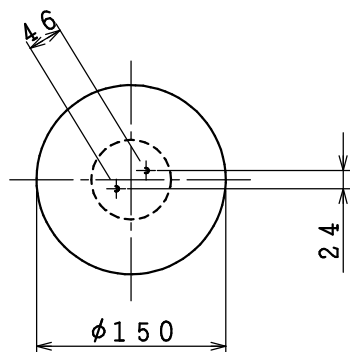
取付寸法(矢視①)
