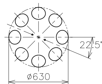
灯具配置/取付角度(下面ヨリ)
