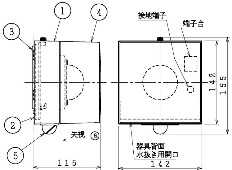
取付寸法 (矢視 (B))
