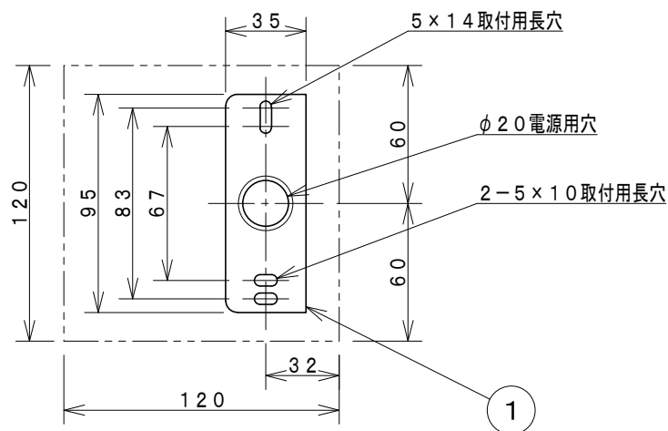
取付寸法 (矢視 a)
