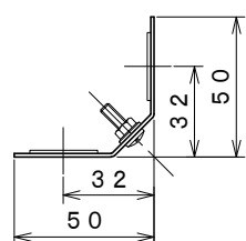
取付寸法 (矢視 a)
