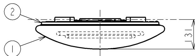
矢視 ㊤
