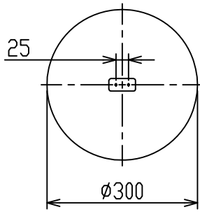
取付寸法(矢視 ①) (S=1/2)
