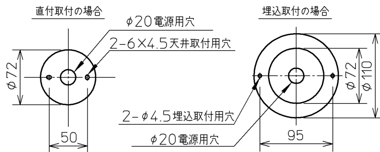
取付寸法（矢視a）
