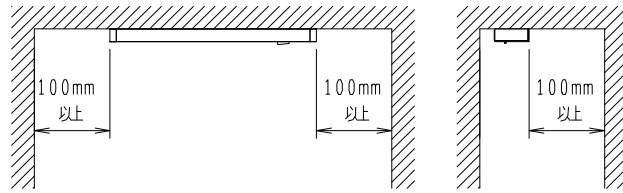
エンドキャップ 着脱必要寸法 S=1/10
