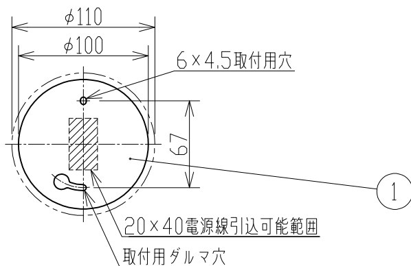
取付寸法(矢視a)
