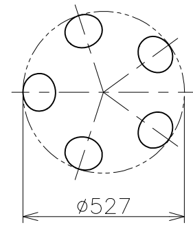
灯具配置図
