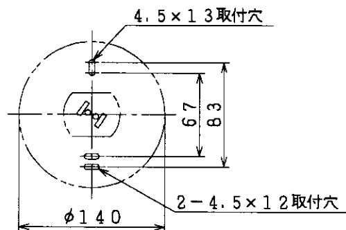
取付寸法（矢視②）
