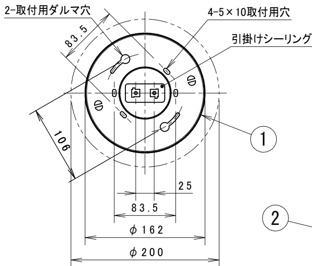
取付寸法(矢視a) (縮尺1/10)
