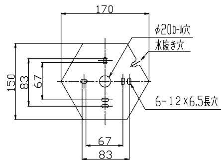
取付寸法（矢視②）
