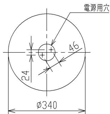
取付寸法(矢視 ㊟)
