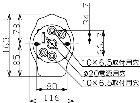
取付寸法 (矢視 ①)
