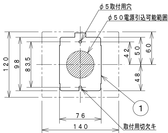
取付寸法 (矢視 a)
