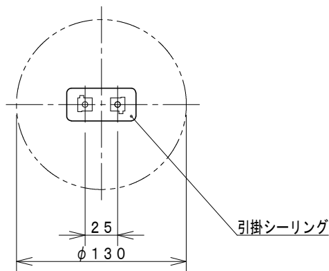
取付寸法 (矢視 a)
