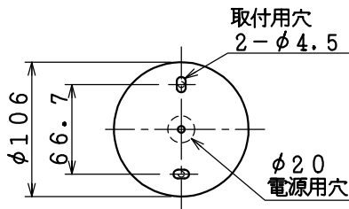
取付寸法(矢視⑧)
