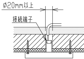
取付寸法(矢視 ②)
