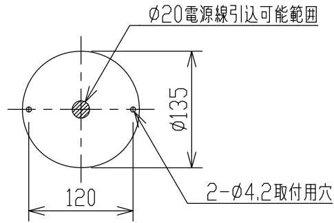
取付寸法(矢視 ②)
