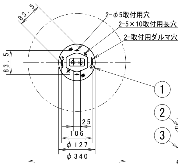
取付寸法(矢視a)
