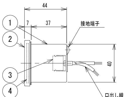
矢視 a ○ →
