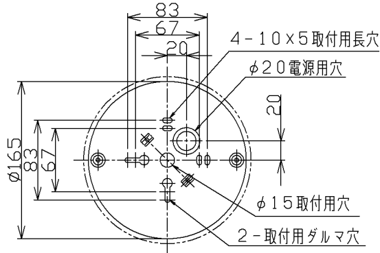
取付寸法 (矢視 ①)
