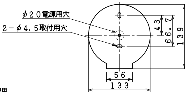
取付寸法(矢視⑧)
