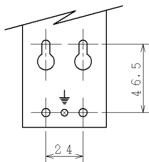
取付寸法 (矢視 ⑧)
