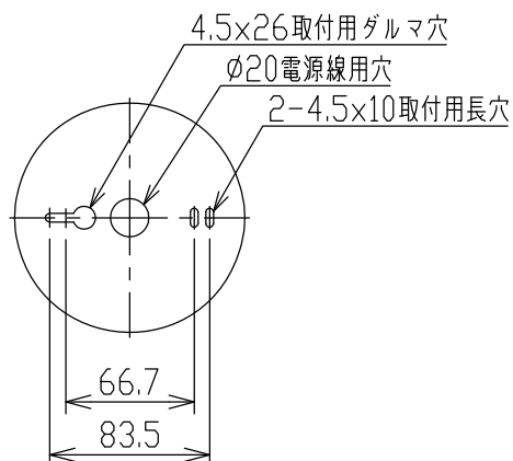
取付寸法(矢視 ②) S=1/2
