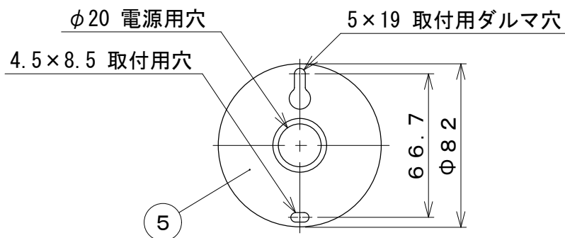
取付寸法 (矢視@)
