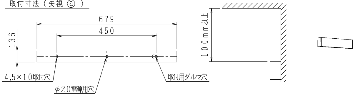
取付寸法（矢視 ②）
