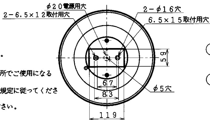
取付寸法（矢視 ㊸）
