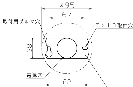
取付寸法（矢視 ①）
