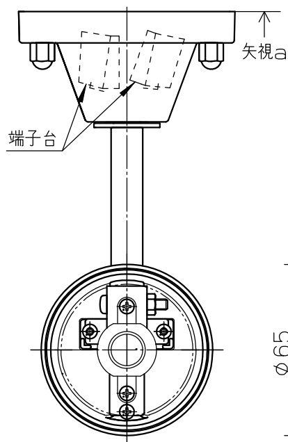
取付寸法 (矢視a)
