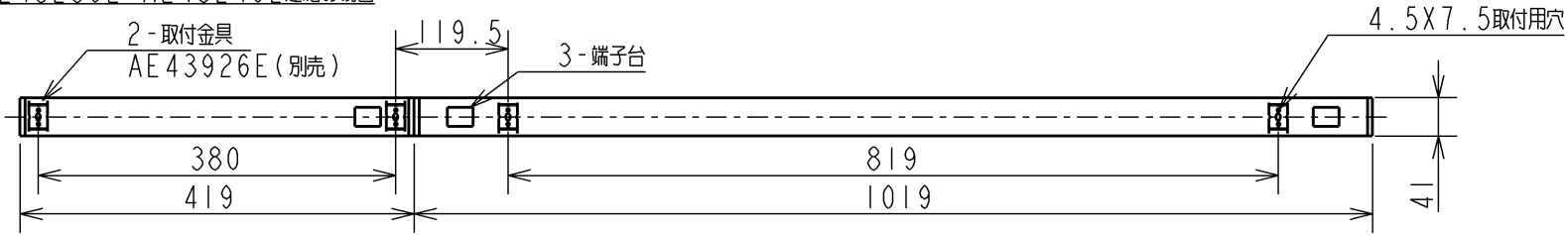
AL43239L+AL43249L 連結の場合
