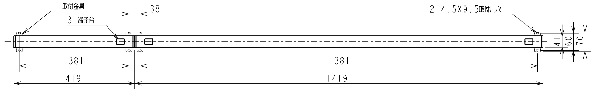
AL 43239L + AL 43259L 連結の場合
