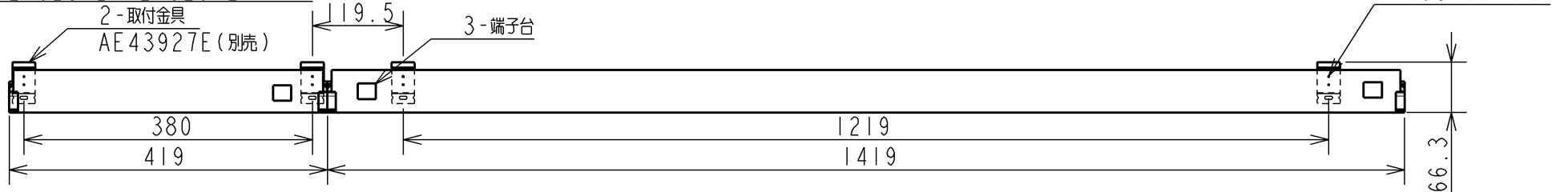
AL43239L+AL43259L 連結の場合
