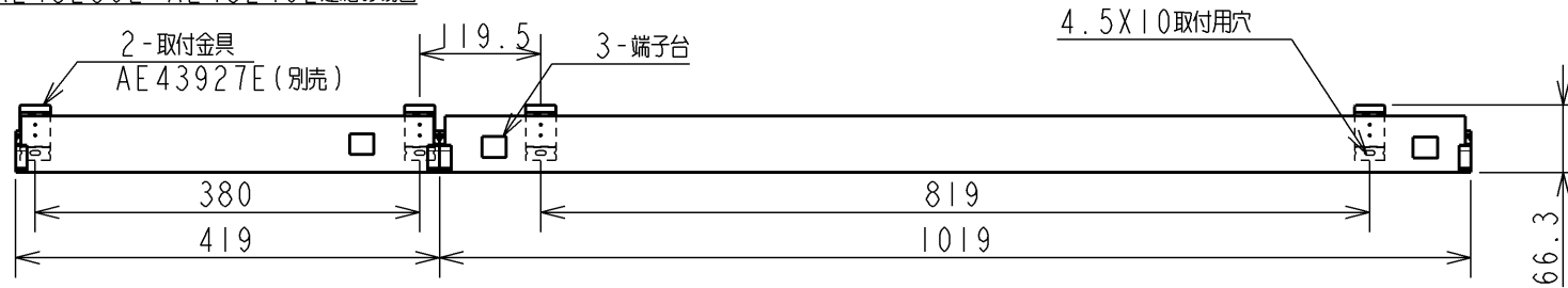
AL43239L+AL43254L 連結の場合
