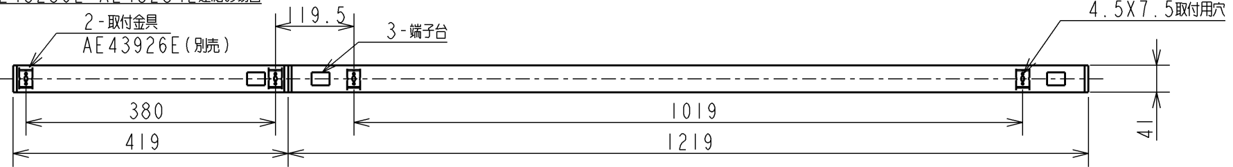
AL43239L+AL43254L 連結の場合
