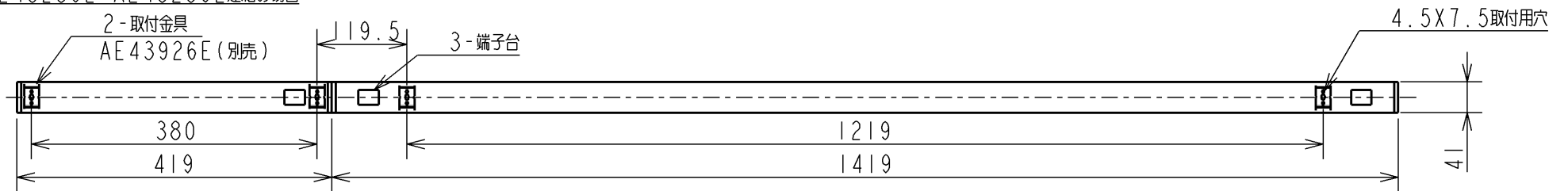
AL43239L+AL43259L 連結の場合
