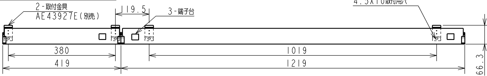
AL43239L+AL43259L 連結の場合
