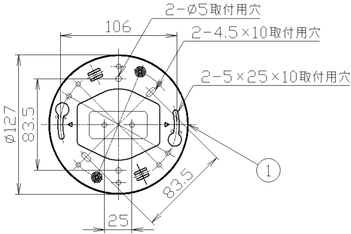
取付寸法 (㊤ 矢視)
