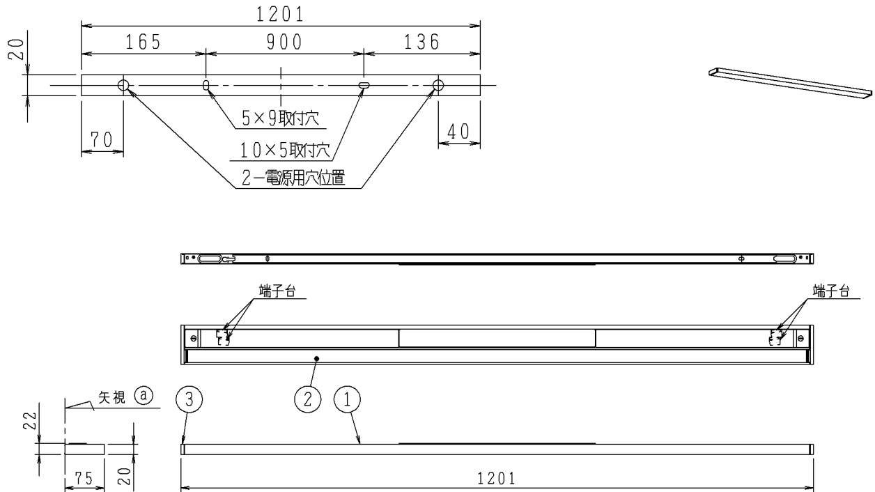
取付寸法（矢視 ①）
