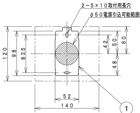
取付寸法 (矢視 a)
